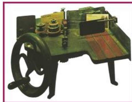
Coll. Musée de La Poste de Caen Machine à oblitérer Krag, 2 e génération 1921-1959
